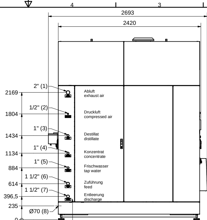
Anschlussblech / connection plate
