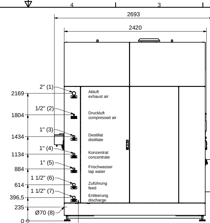
Anschlussblech / connection plate
